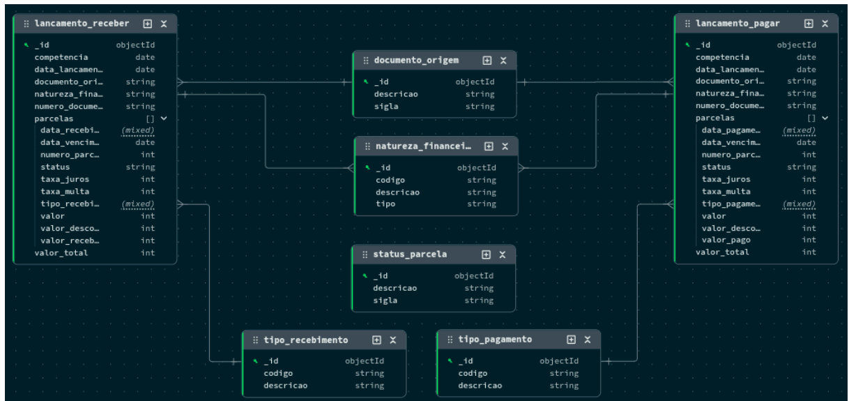
Figura 1 - Modelo Lógico Banco de Dados ERP Financeiro
